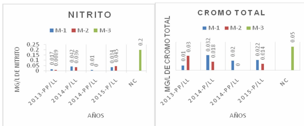
Figura 9. Comportamiento del nitrito y cromo total.
