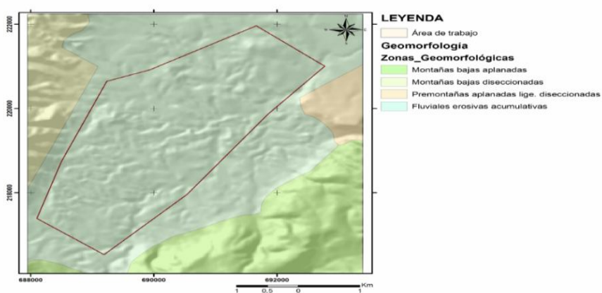
Figura 3. Mapa geomorfológico del área de estudio (modificado de Rodríguez A, 1999)
