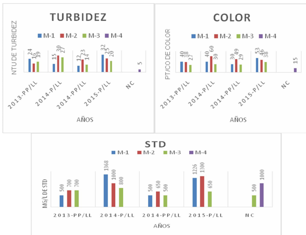
Figura 6. Comportamiento de la turbidez, color y sólidos totales disueltos (STD).
