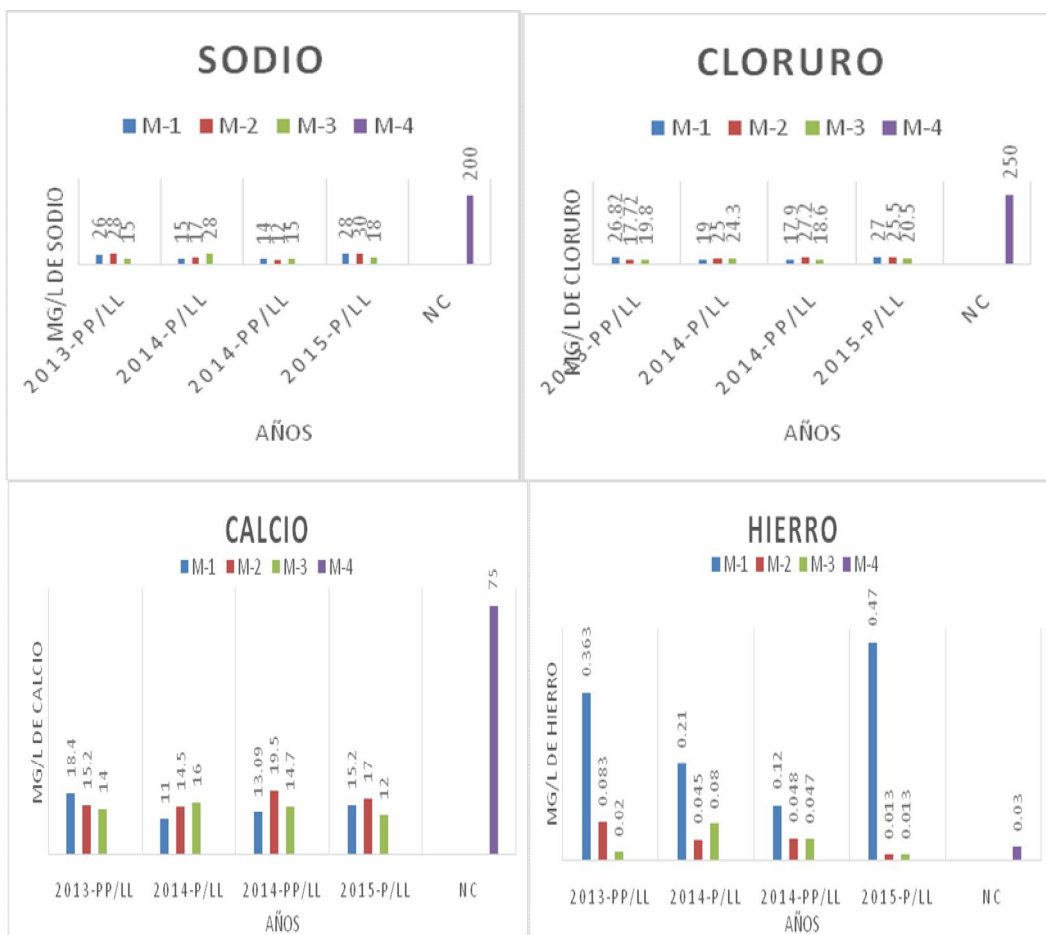
Figura 7. Comportamiento del sodio, cloruro, calcio y hierro.
