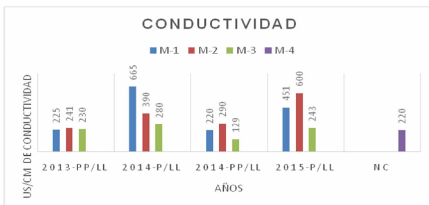
Figura 5. Comportamiento de la conductividad eléctrica.
