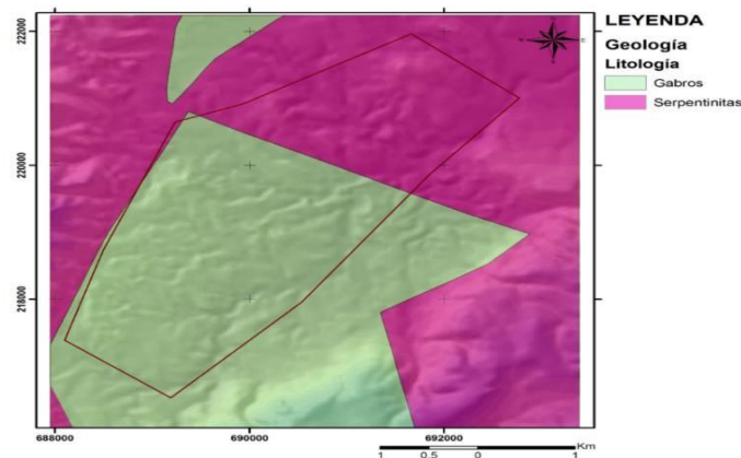
Figura 4. Mapa geológico del área de estudio (modificado de Rodríguez A, 1999)
