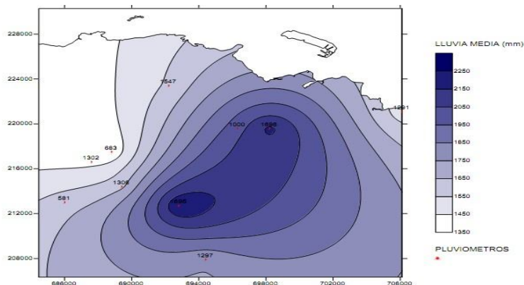
Figura 2. Mapa pluviométrico del territorio de Moa. Escala 1:50 000 (Instituto Nacional de Recursos Hidráulicos, Habana, 2005) (tomado de Ramírez Y, 2010)
